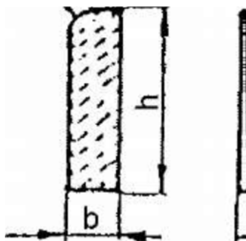
Rysunek 1. Kształt betonowego obrzeża chodnikowego
