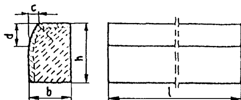
Rys. 1. Wymiarowanie krawężników
