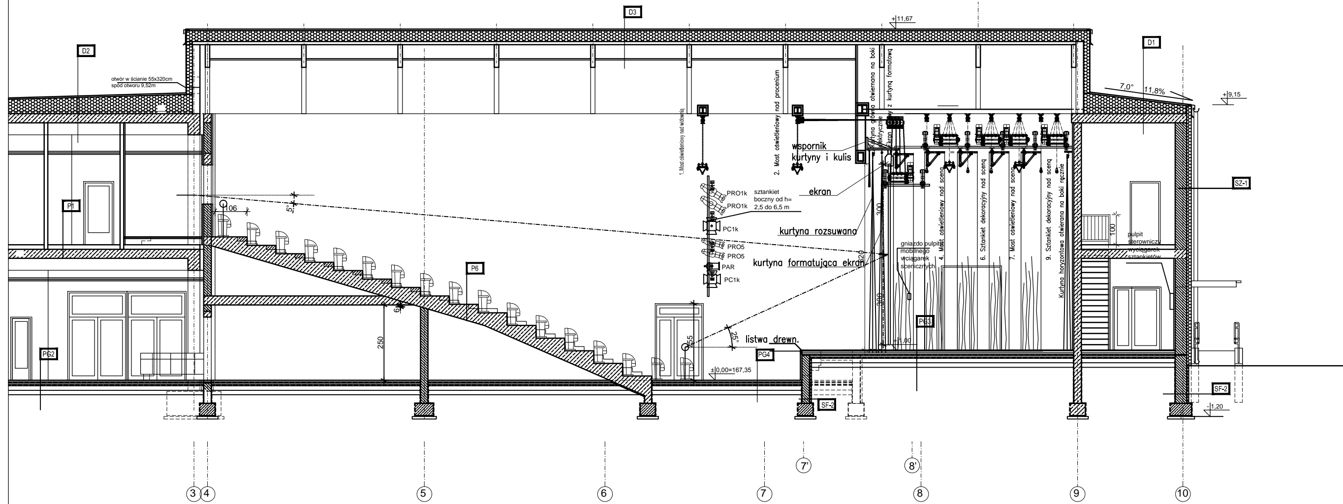
przekrój I a - I a
