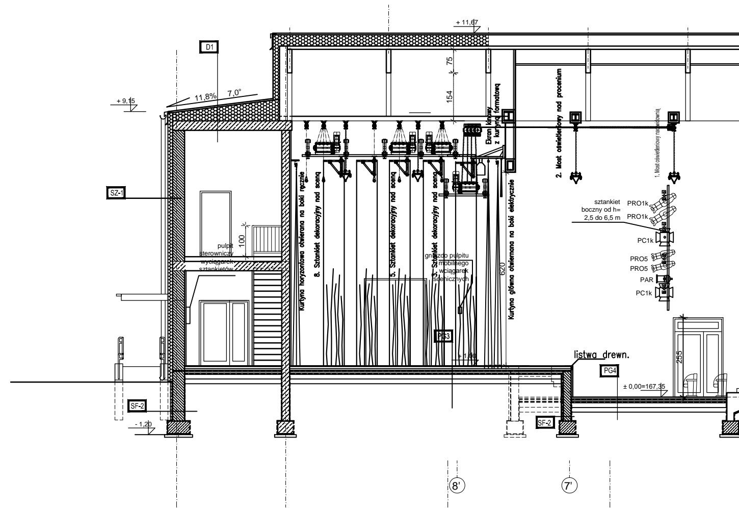
przekrój I b - I b
